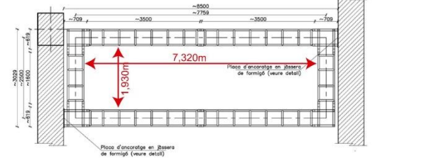
PLANTA SUPERIOR
