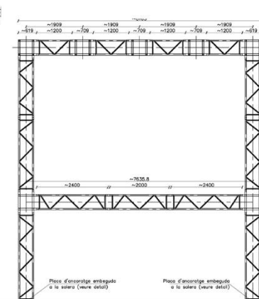
SECCIÓ TRANSVERSAL
