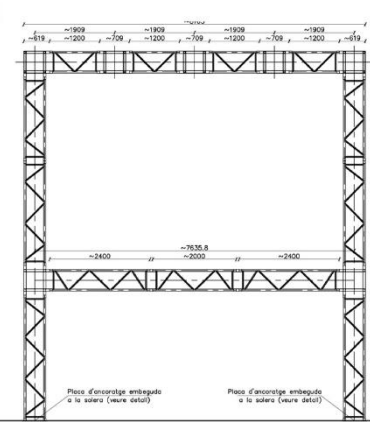
SECCIÓ TRANSVERSAL
