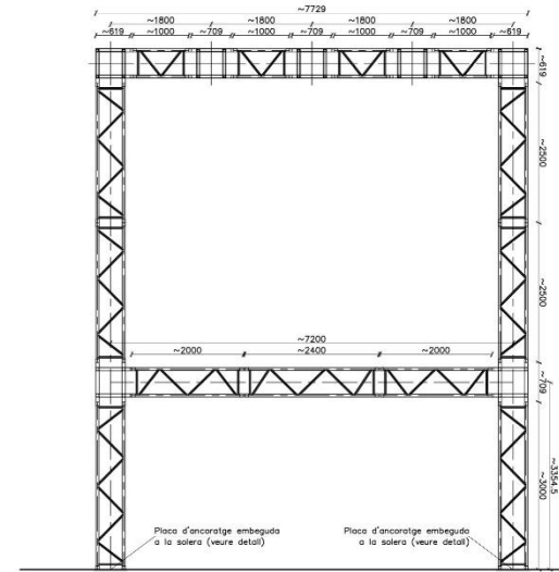
SECCIÓ TRANSVERSAL
