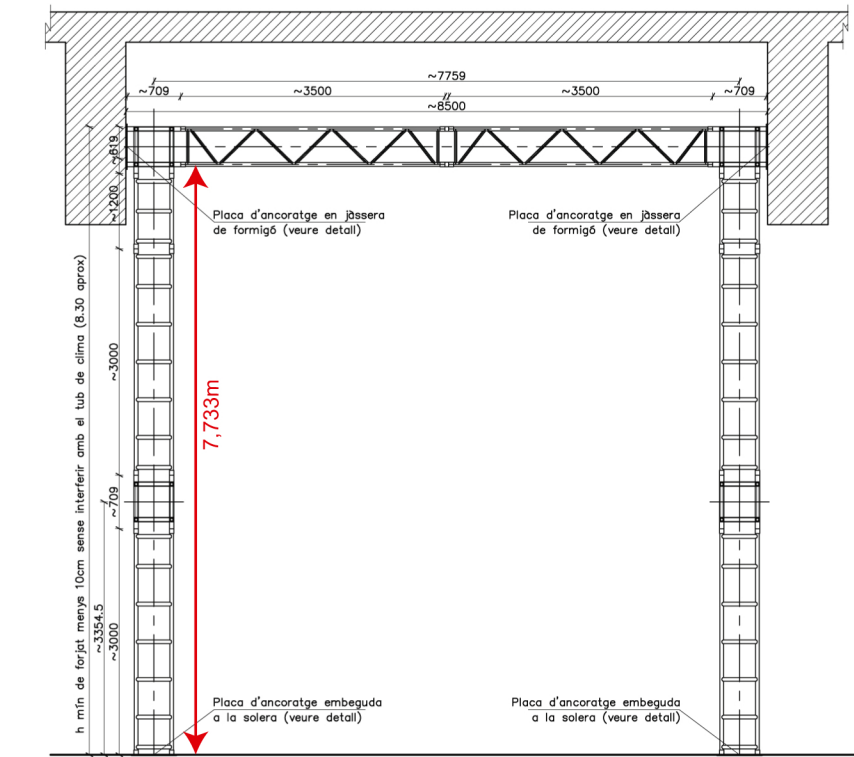
SECCIÓ LONGITUDINAL
