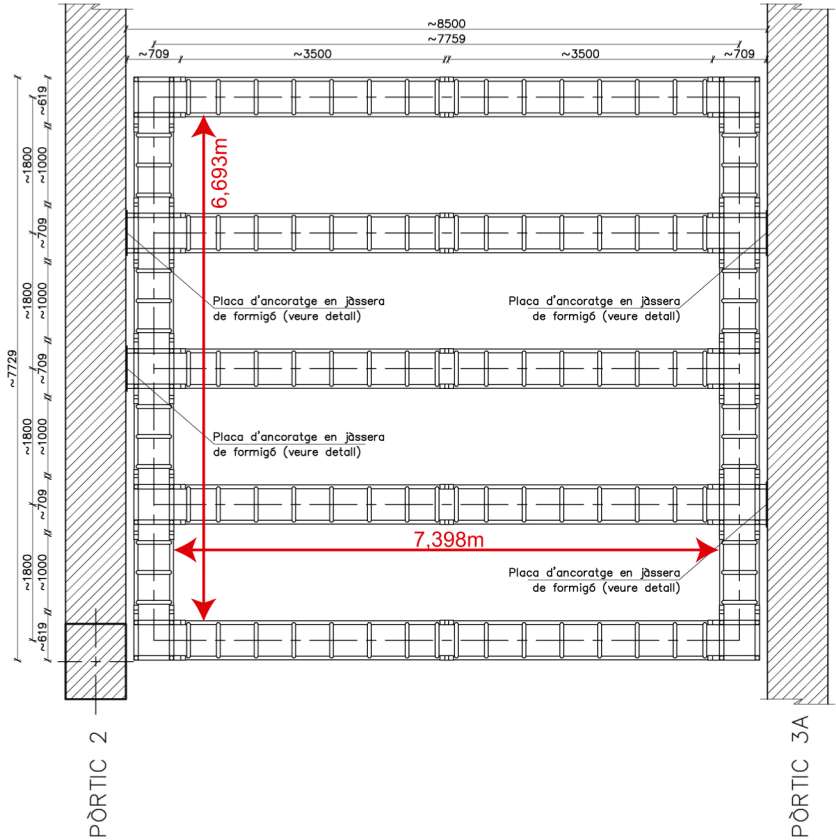
PLANTA SUPERIOR
