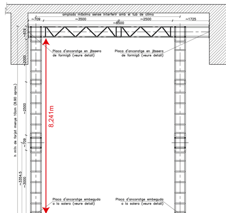
SECCIÓ LONGITUDINAL
