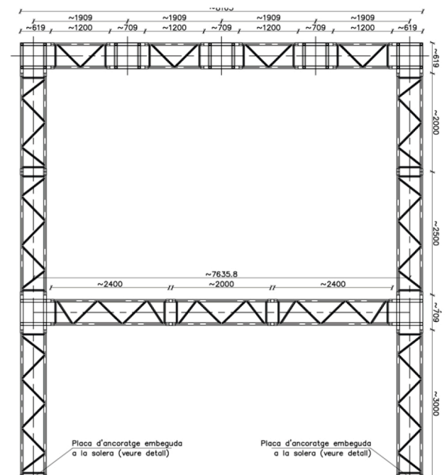
SECCIÓ TRANSVERSAL
