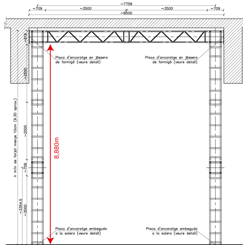
SECCIÓ LONGITUDINAL
