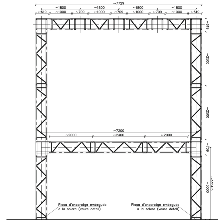
SECCIÓ TRANSVERSAL
