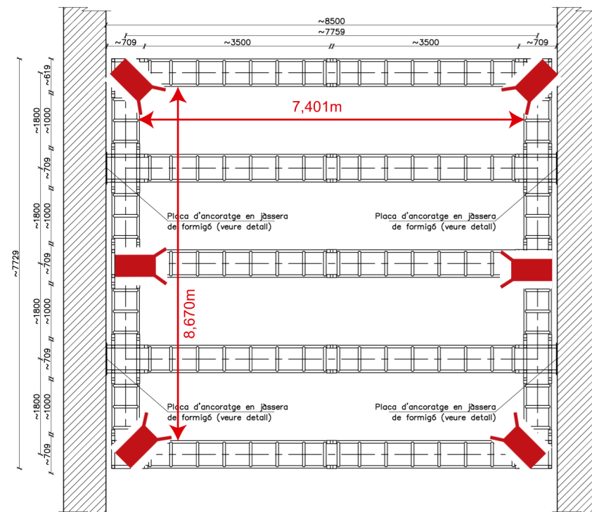
PLANTA SUPERIOR
